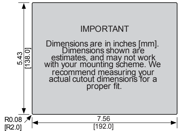
Cutout Dimensions
