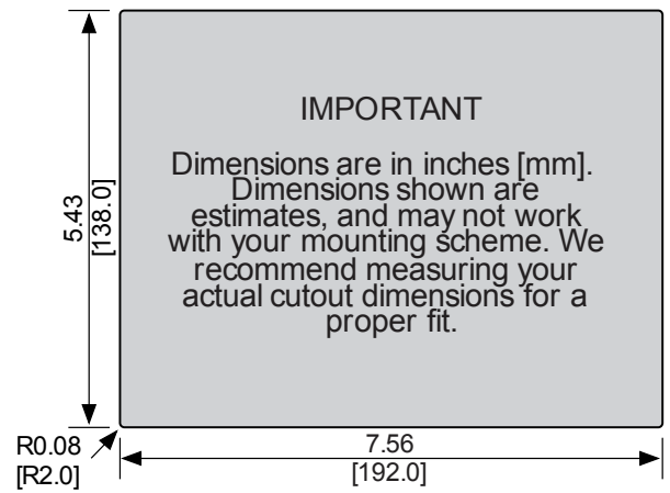
Cutout Dimensions
