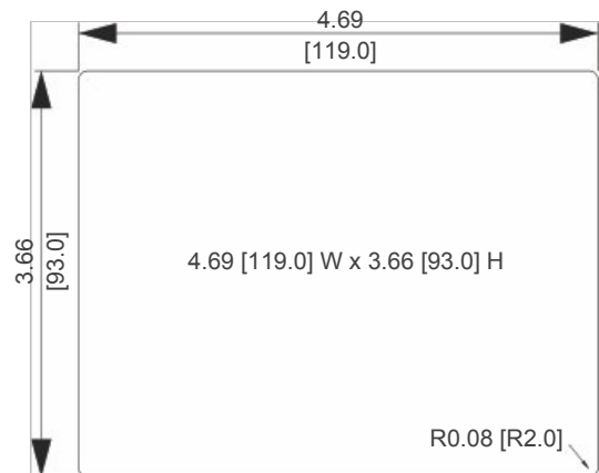
Cutout Dimensions
